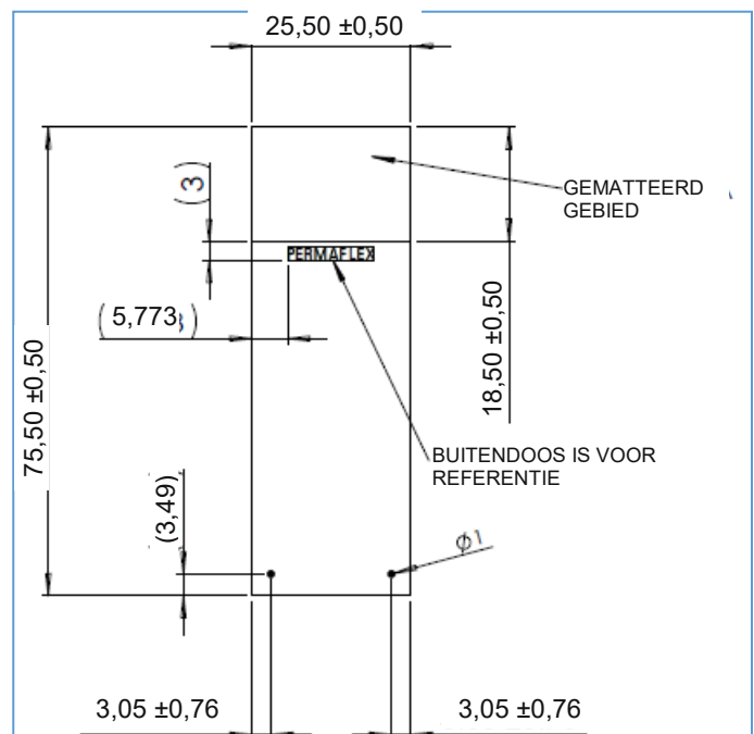
PERMAFLEX™ microglaasje tekening, mm
